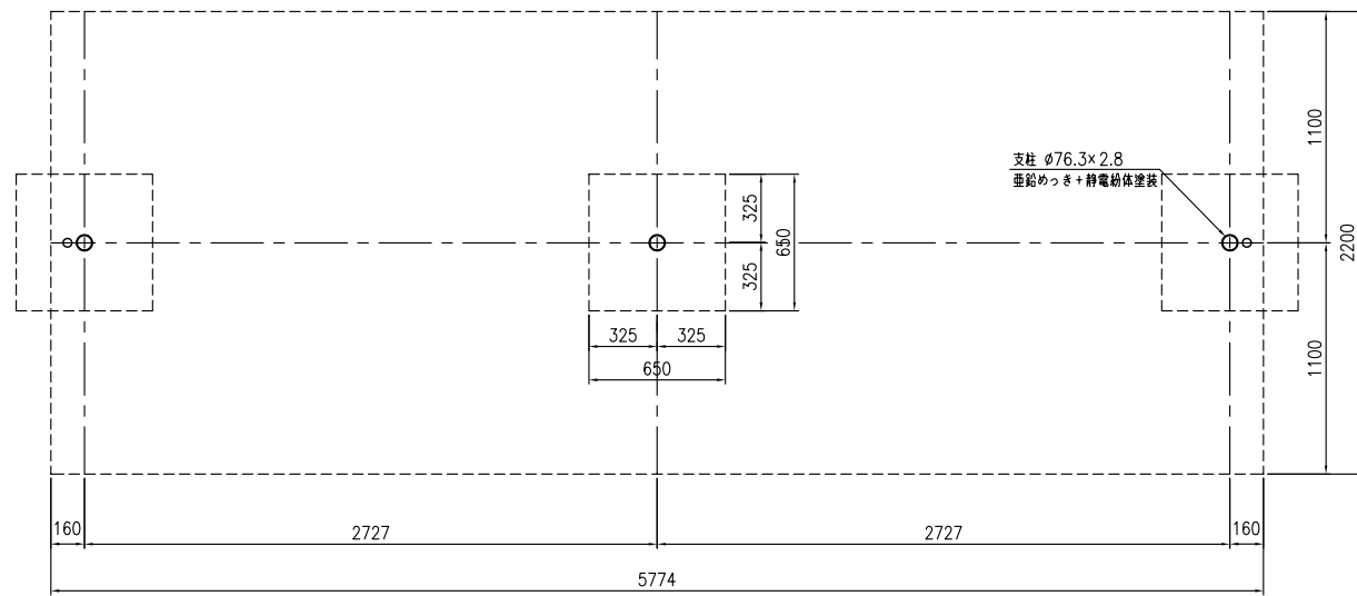
平面図 (S=1:20) (▼印: 縦断とし位置)
