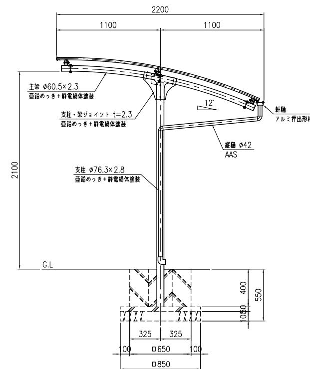
側面図 (S=1:20)
