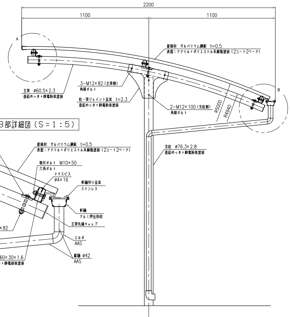
断面図 (S=1:10)
