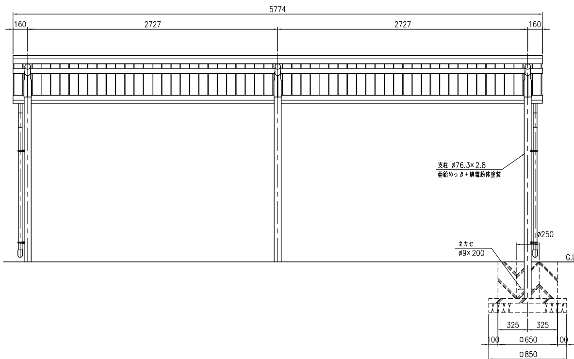
正面図 (S=1:20)
