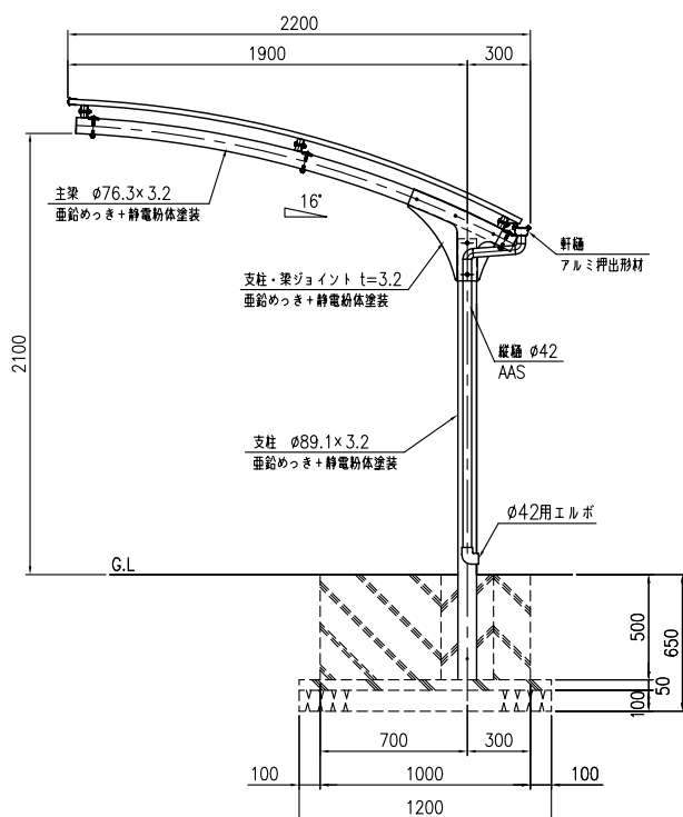
側面図 (S=1:20)
