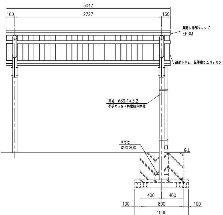
正面図 (S=1:20)
