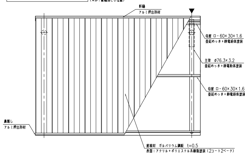
正面図 (S=1:20)
