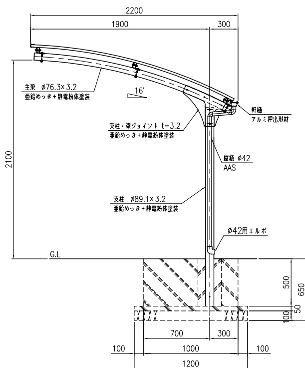
側面図 (S=1:20)
