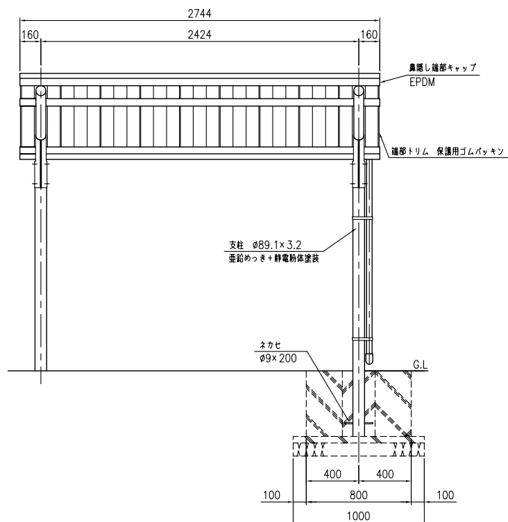
正面図 (S=1:20)
