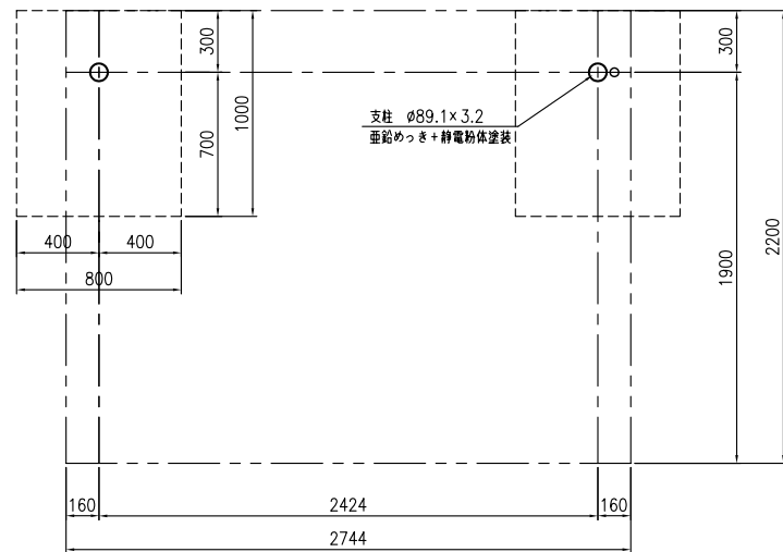
基礎伏図 (S=1:20)
