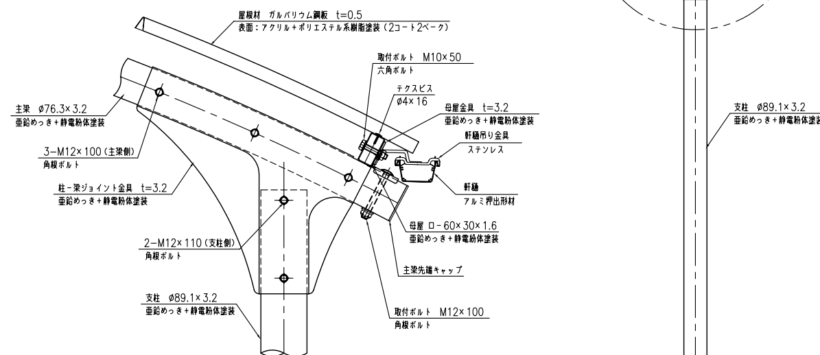
B部詳細図 (S=1:5)
