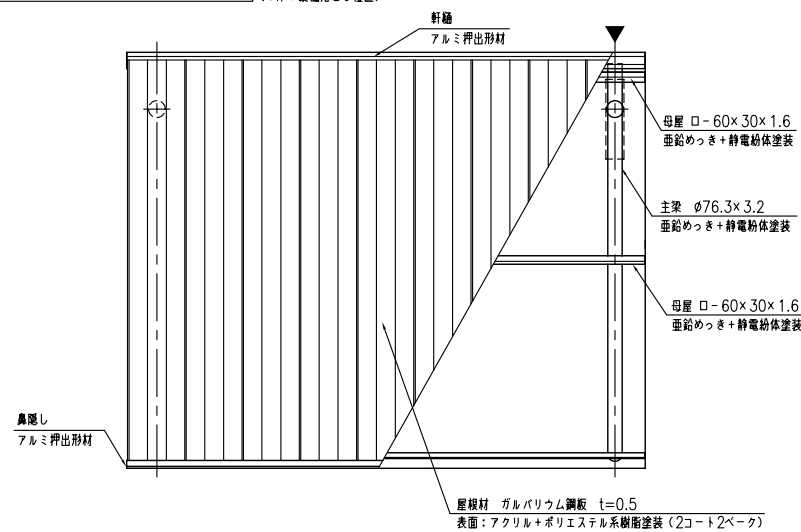
正面図 (S=1:20)
